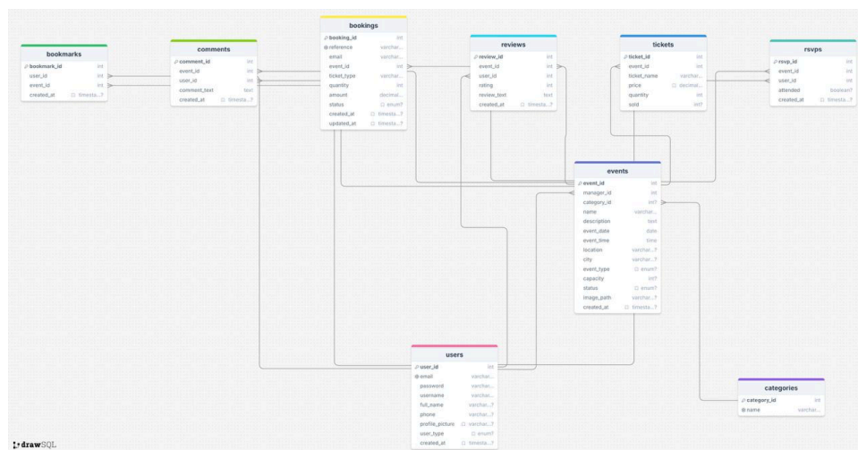
ER diagram
